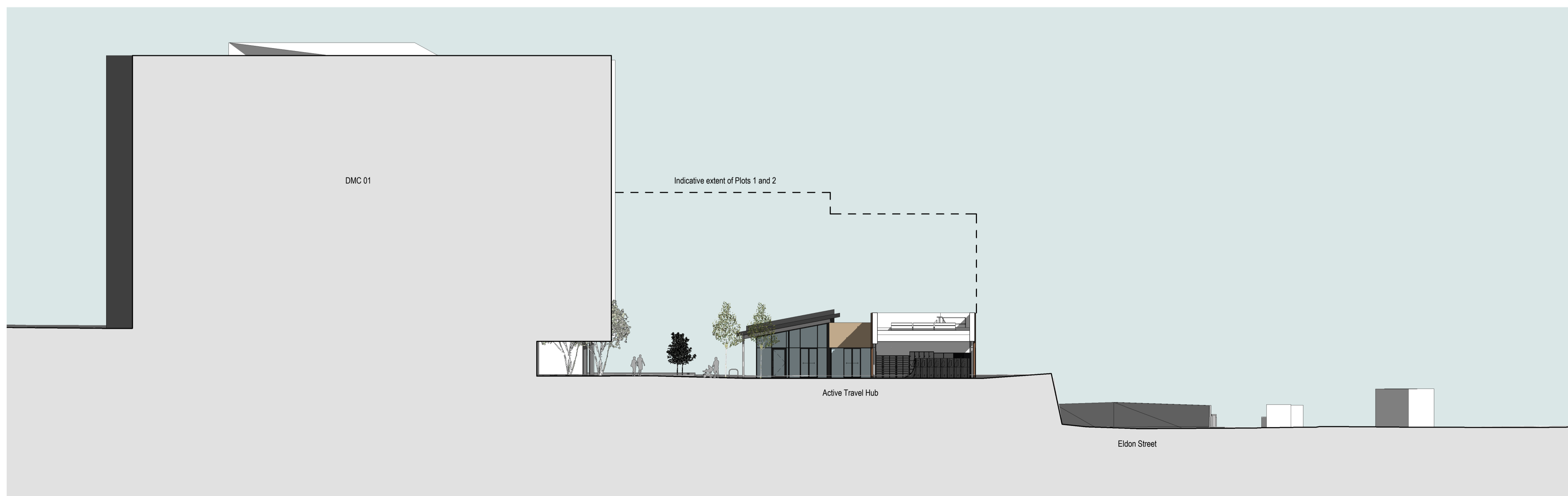
2 ATH Cross Section 2 1 : 200
