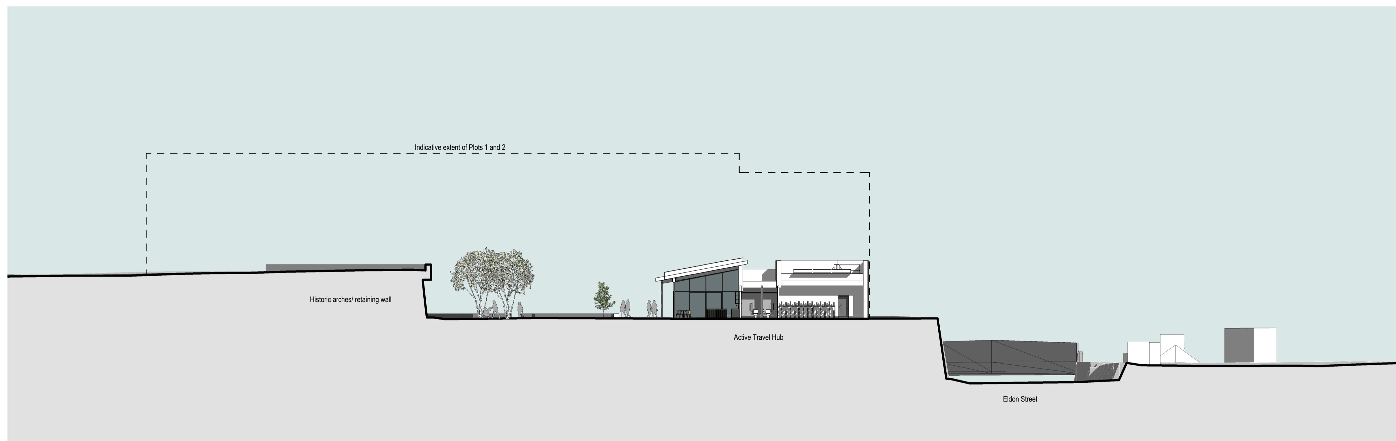
1 ATH Site Cross Section 1 1 : 200
