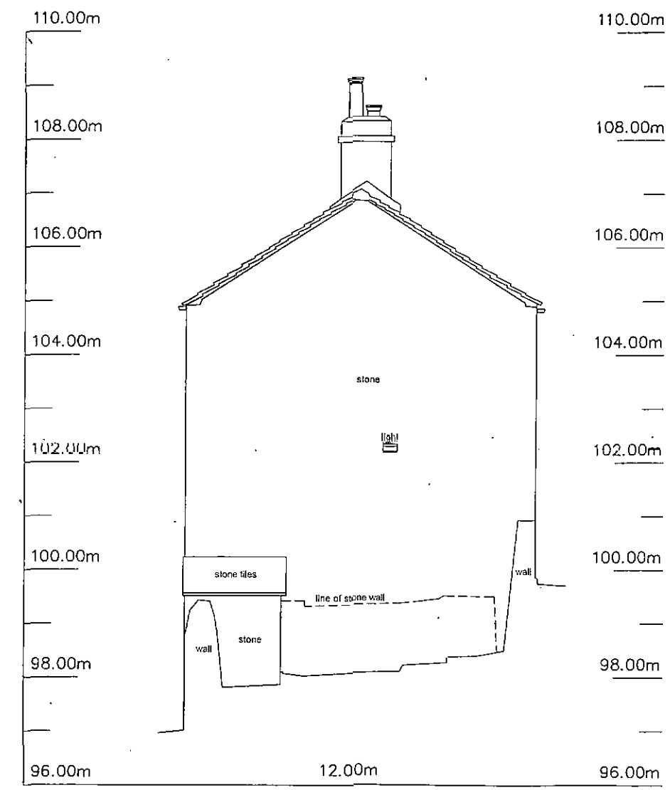
ELEVATION D-D
