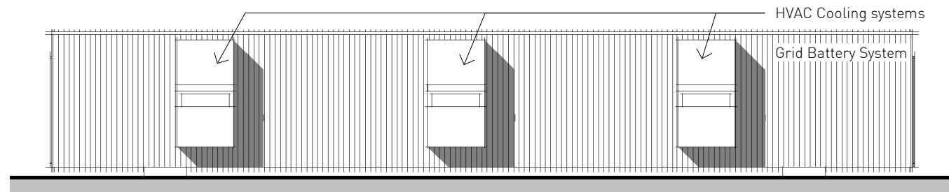
ELEVATION 1 1 : 100
