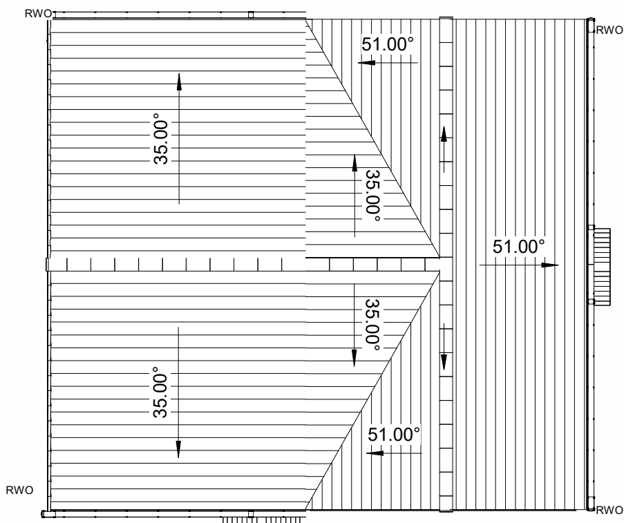
Roof Plan 1 : 100
