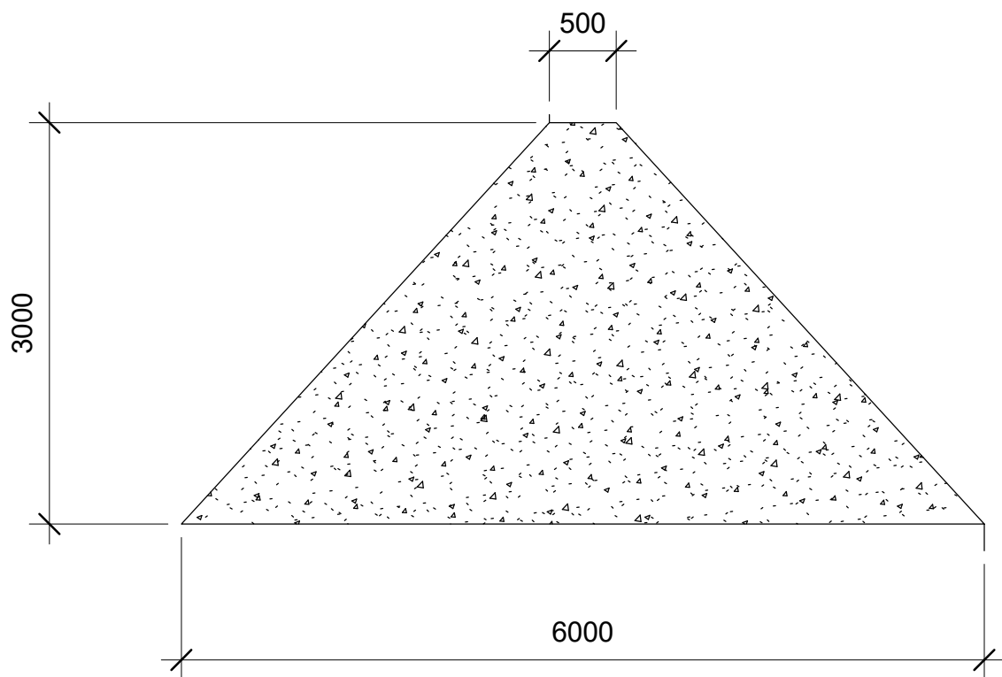
1 Bund Section 1 : 50
