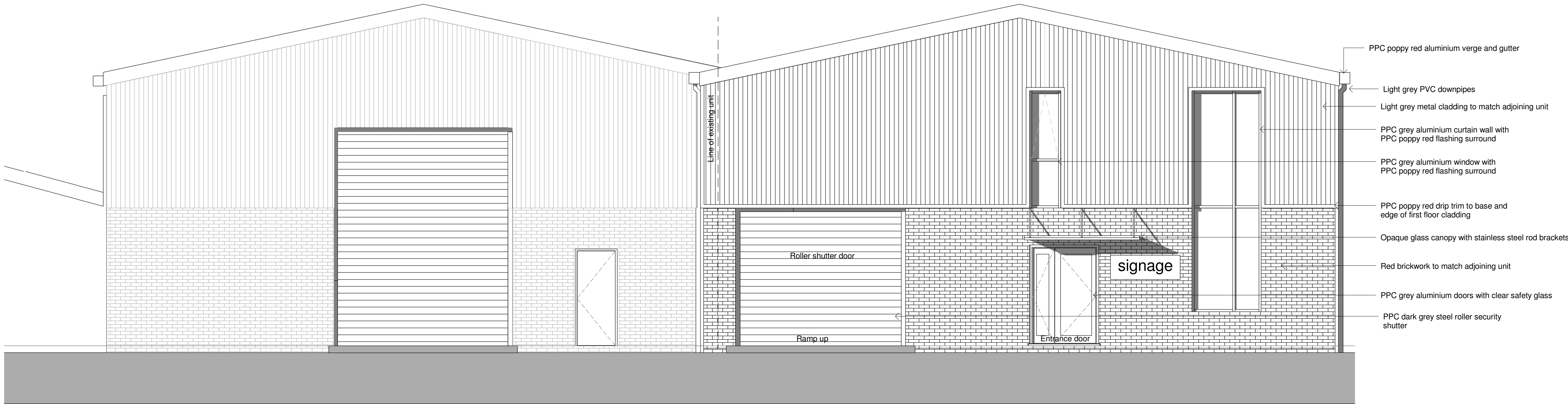
1 Elevation 1 - a 1 : 50
