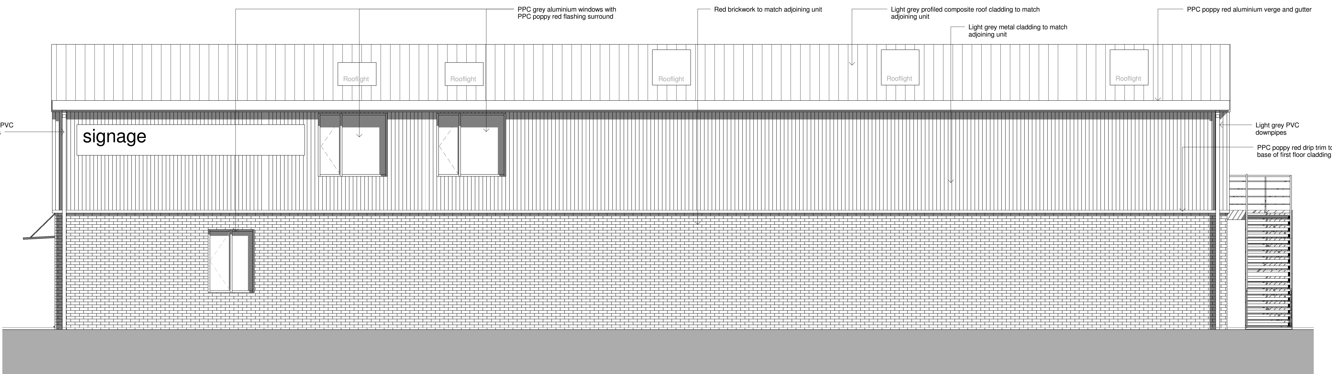
2 Elevation 2 - a 1 : 50
