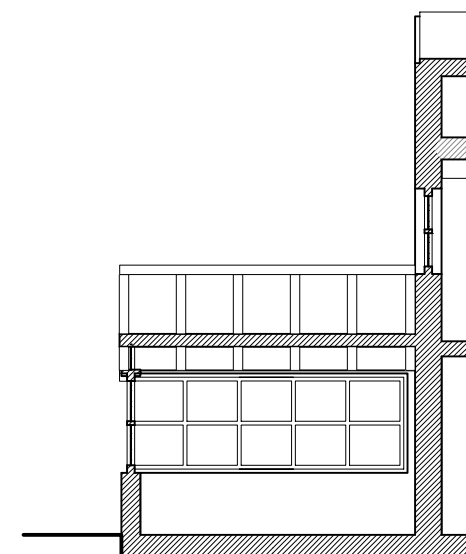
4 Existing Section Scale: 1:100
