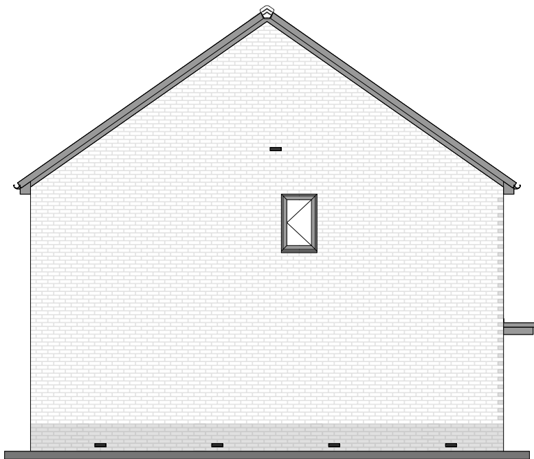
RIGHT ELEVATION
