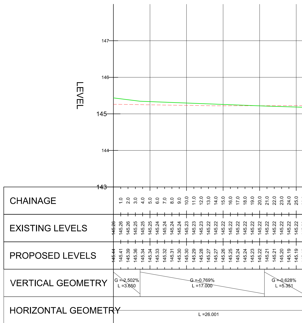
RD-02 - LONGSECTION SCALE: H 1:250,V 1:50. DATUM: 143.000
