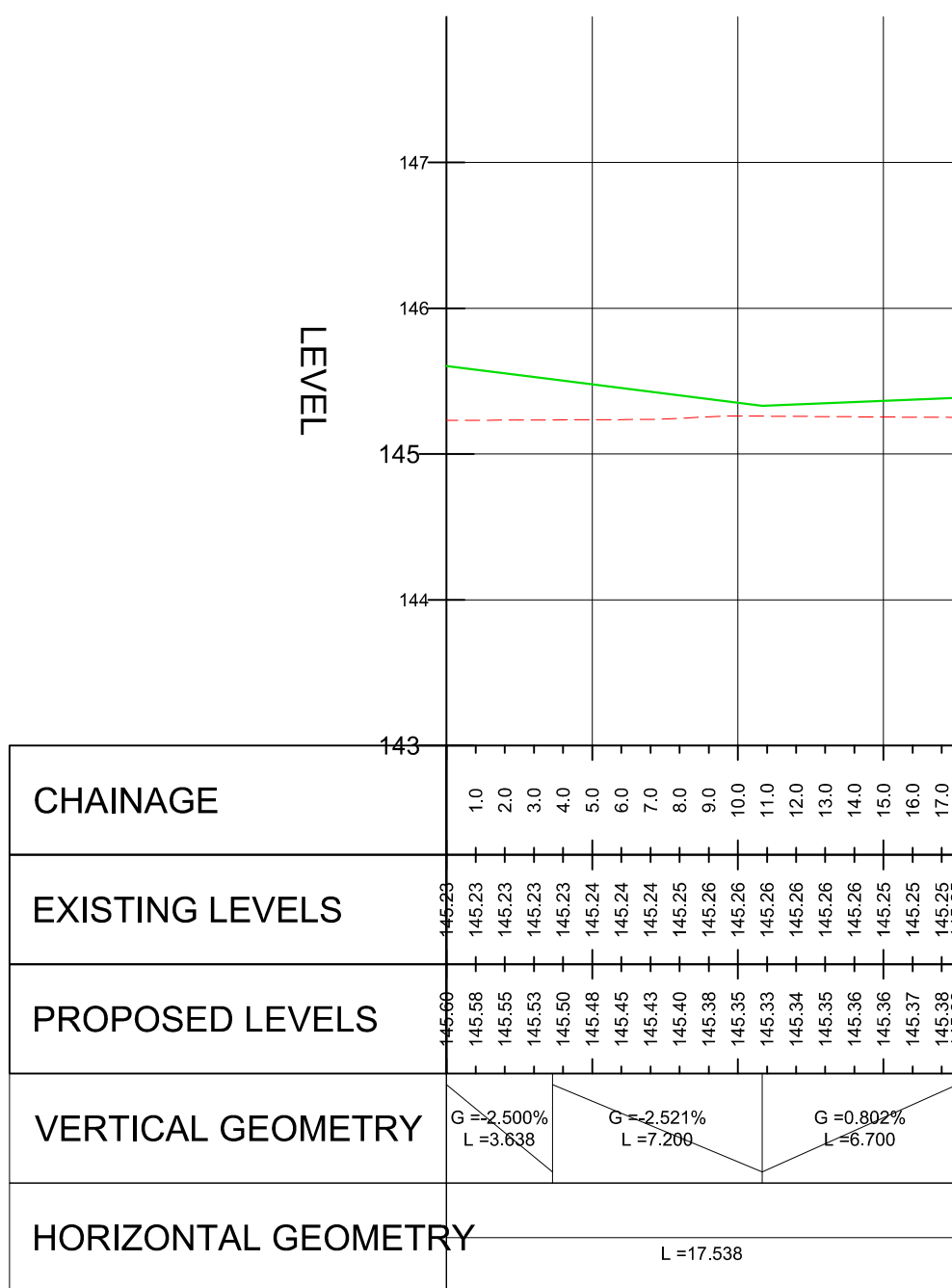
RD-03 - LONGSECTION SCALE: H 1:250,V 1:50. DATUM: 143.000
