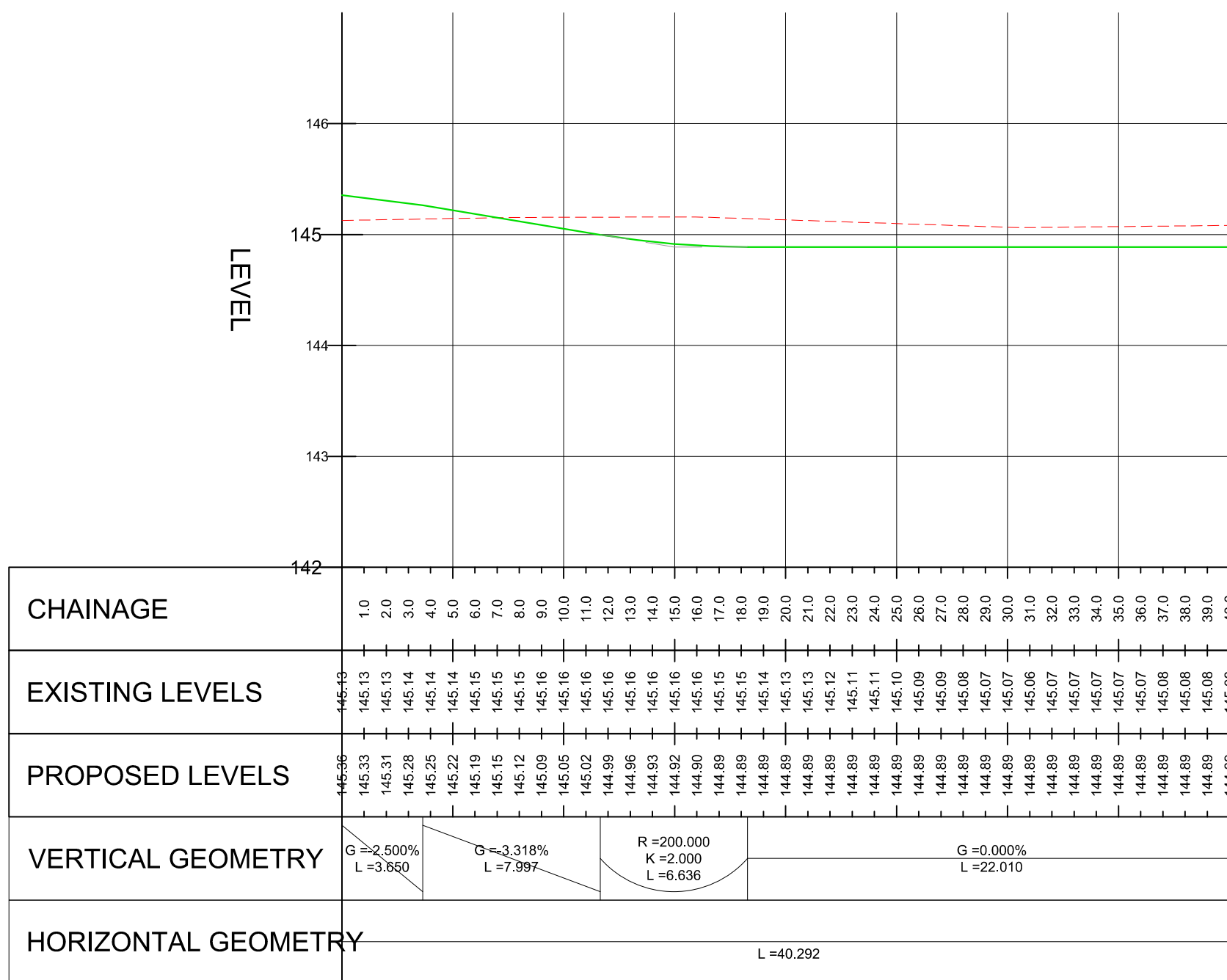
RD-04 - LONGSECTION SCALE: H 1:250,V 1:50. DATUM: 142.000
