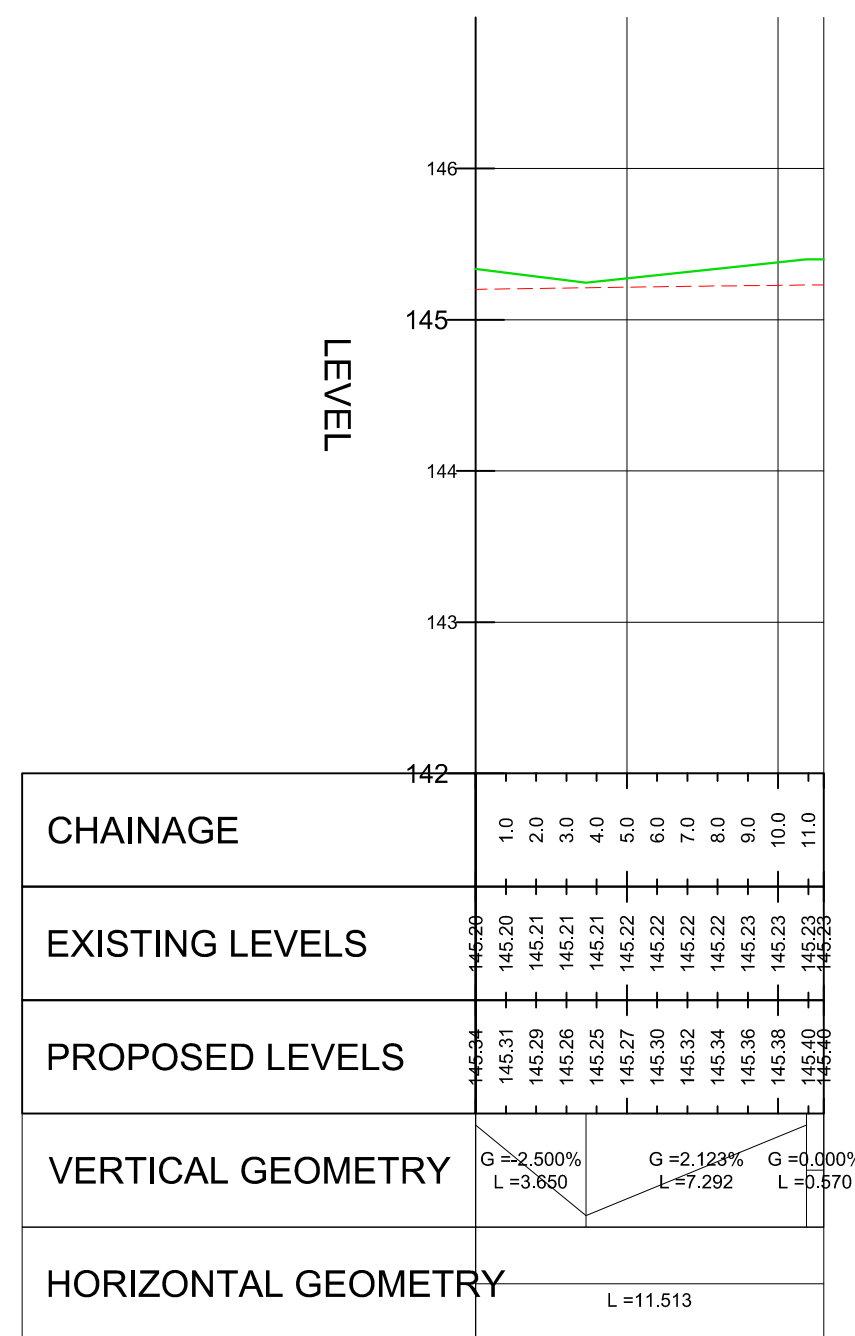
RD-05 - LONGSECTION SCALE: H 1:250,V 1:50. DATUM: 142.000
