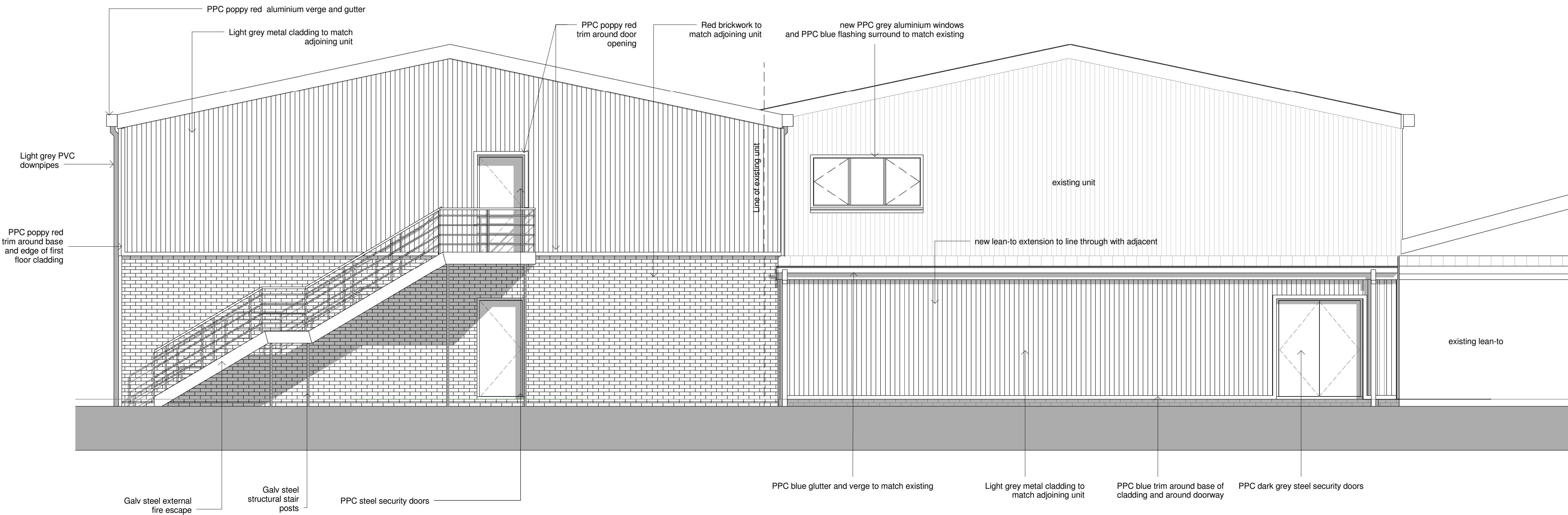
1 Elevation 3 - a 1 : 50
