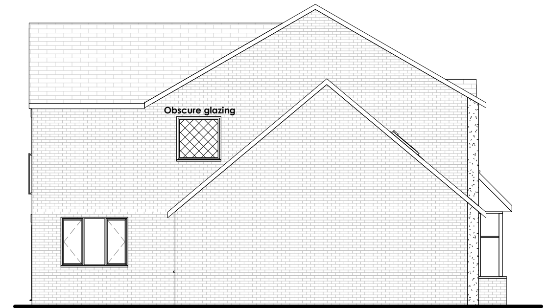
RIGHT ELEVATION 1 : 100
