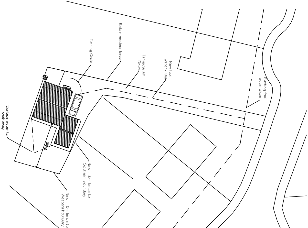
P R O P O S E D S I T E P L A N 1 : 2 0 0
