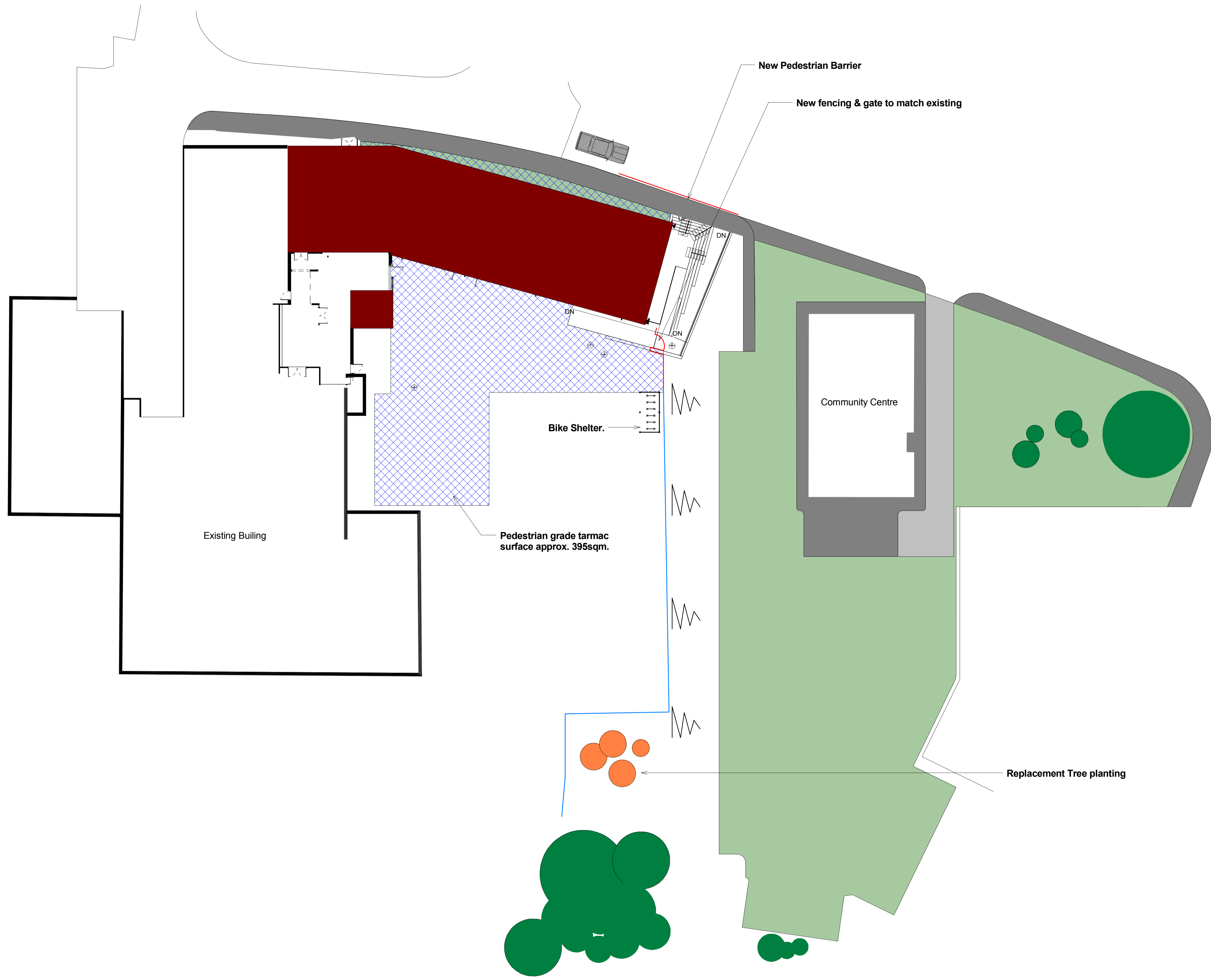
1 Site Works Plan 1 : 200
