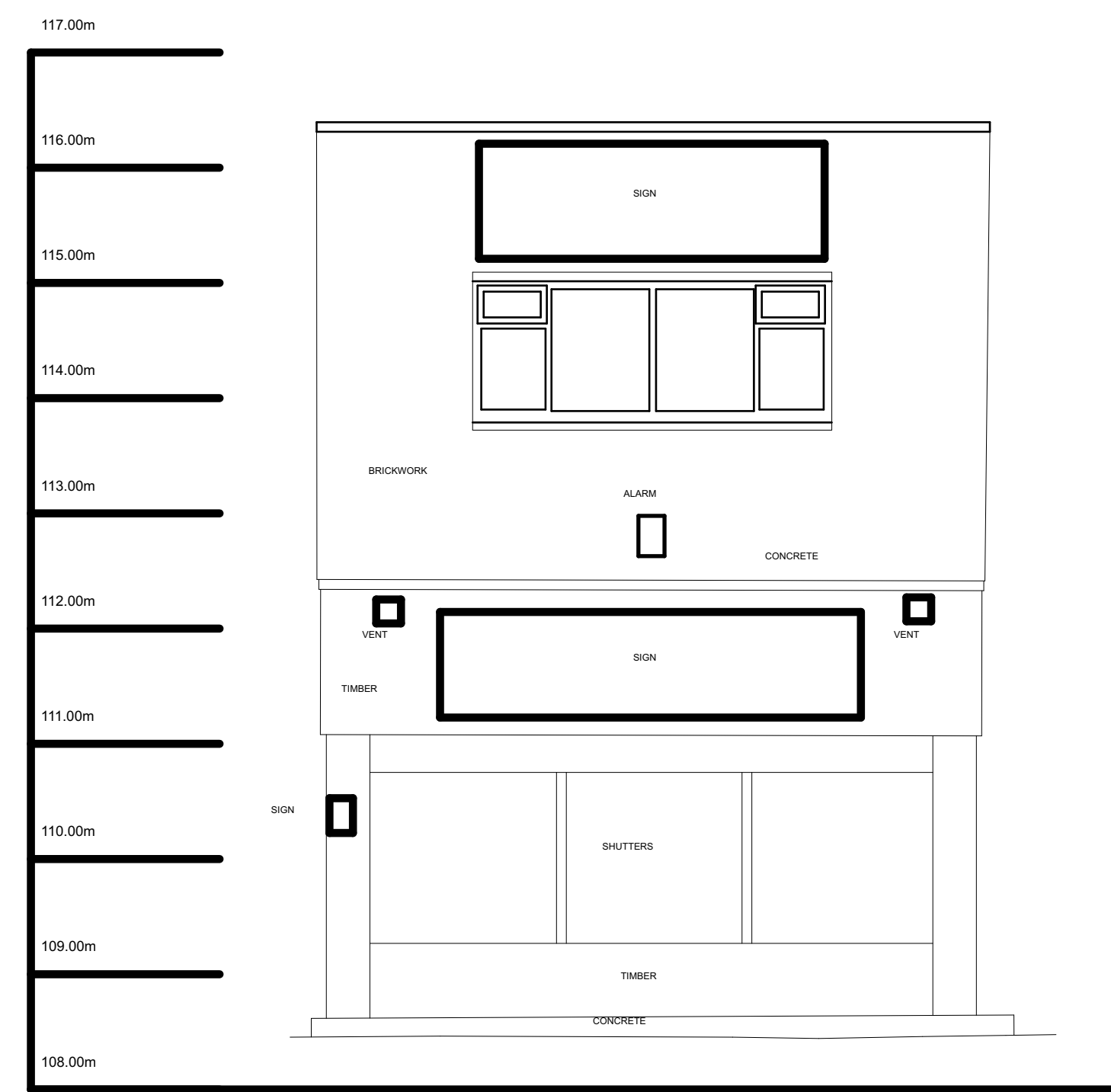
ELEVATION 7
