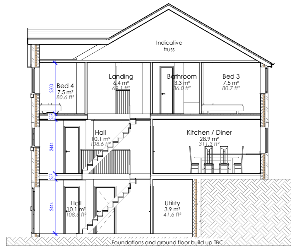
8 | HTE3 Section 1 : 100
