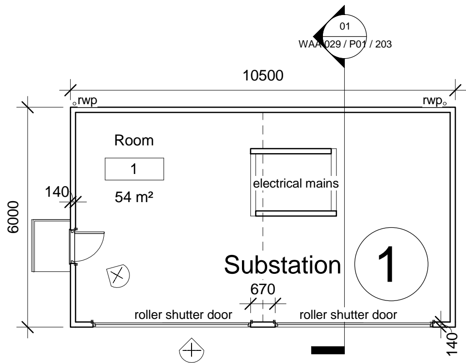
1 Plan Level 1 1 : 100
