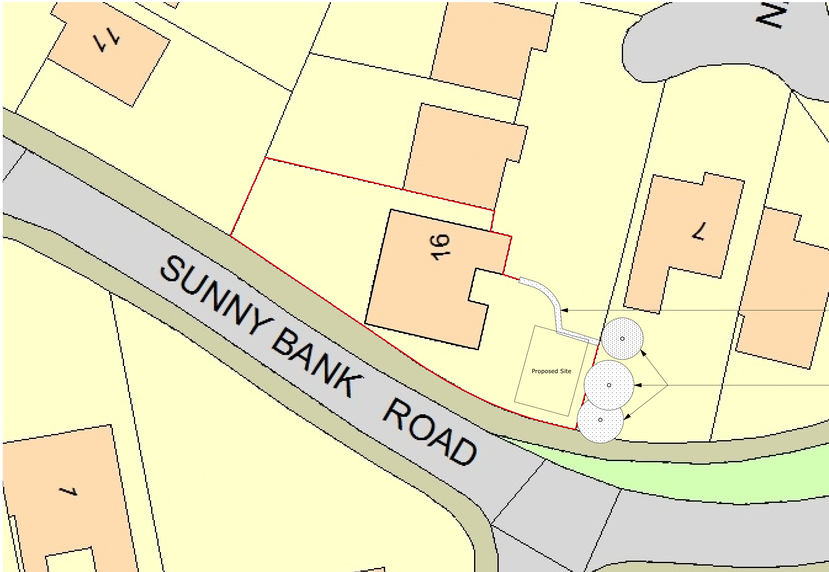
1 Existing Landscape Plan Scale: 1:200
