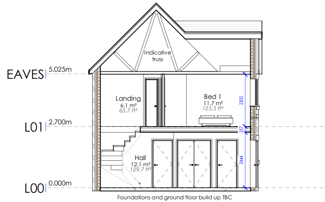
7 | HTG Var Section 1 : 100
