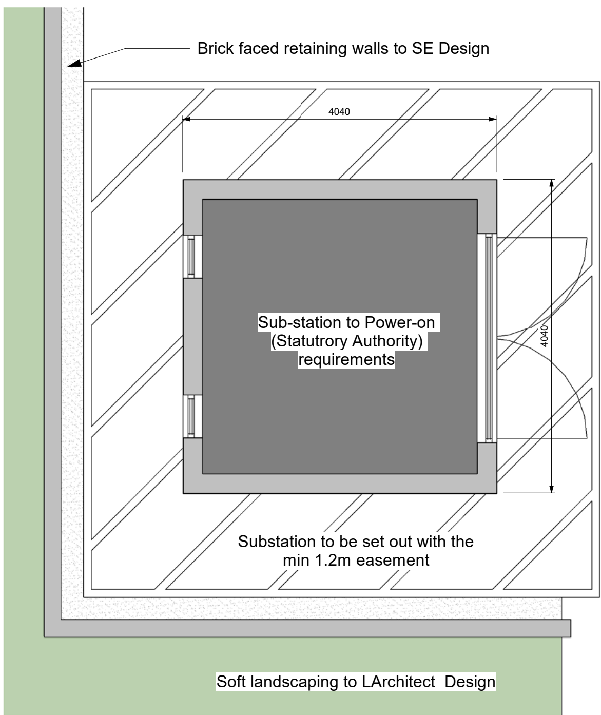
Siteplan - Substation Layout 1 : 50
