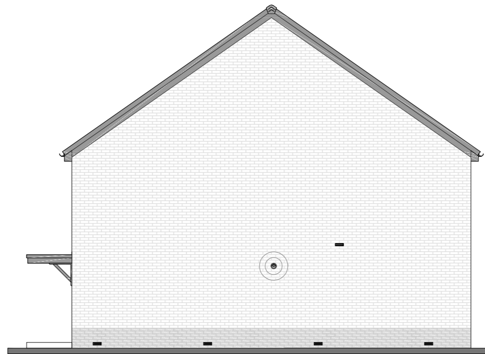
RIGHT ELEVATION
