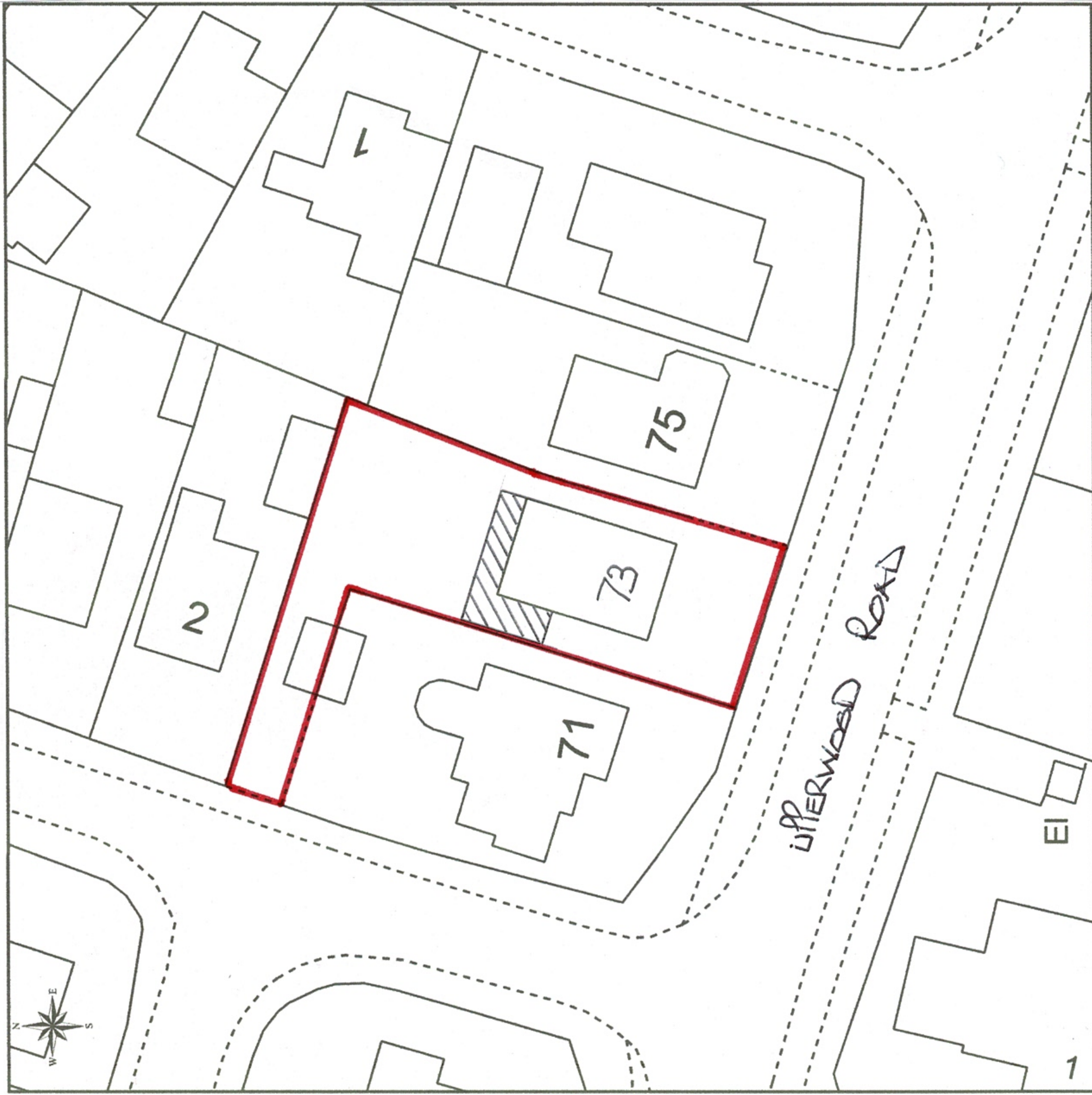
SITE PLAN (1:500)
