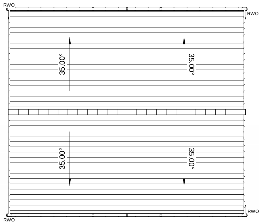
Roof Plan 1 : 100
