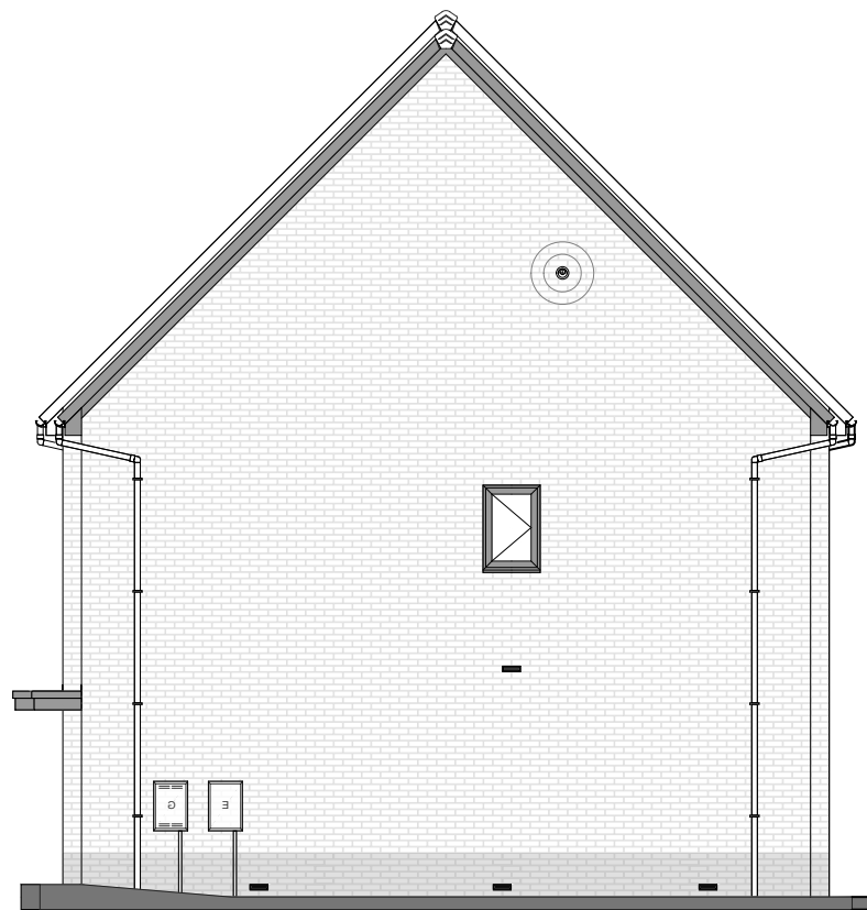
RIGHT ELEVATION
