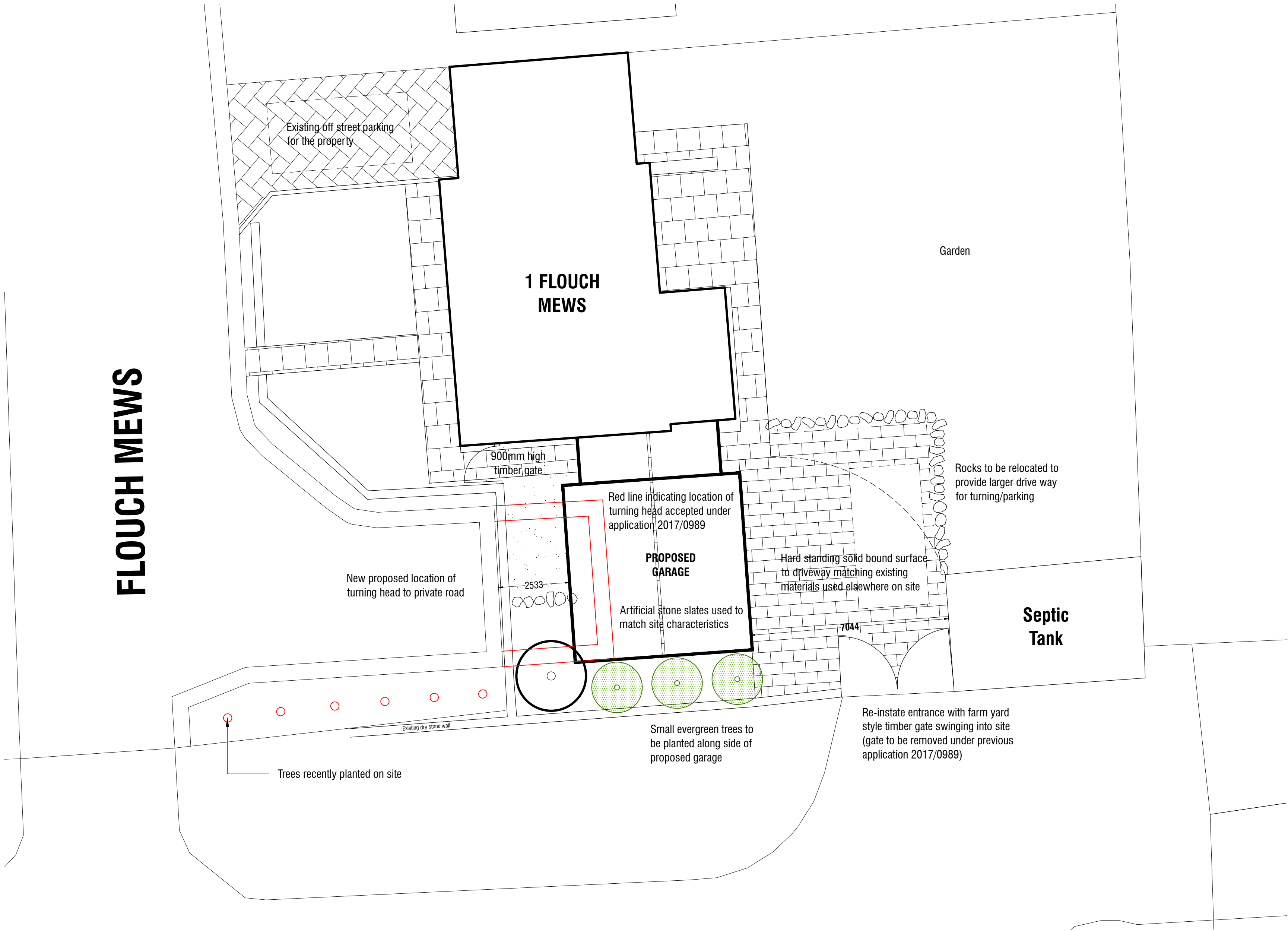
SITE PLAN 1:100
