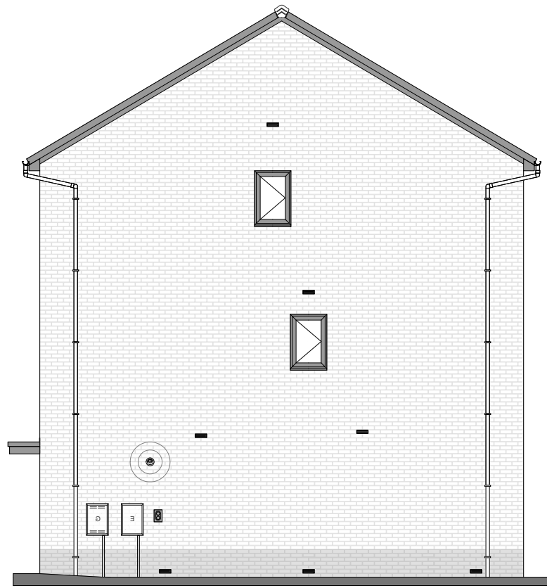
RIGHT ELEVATION
