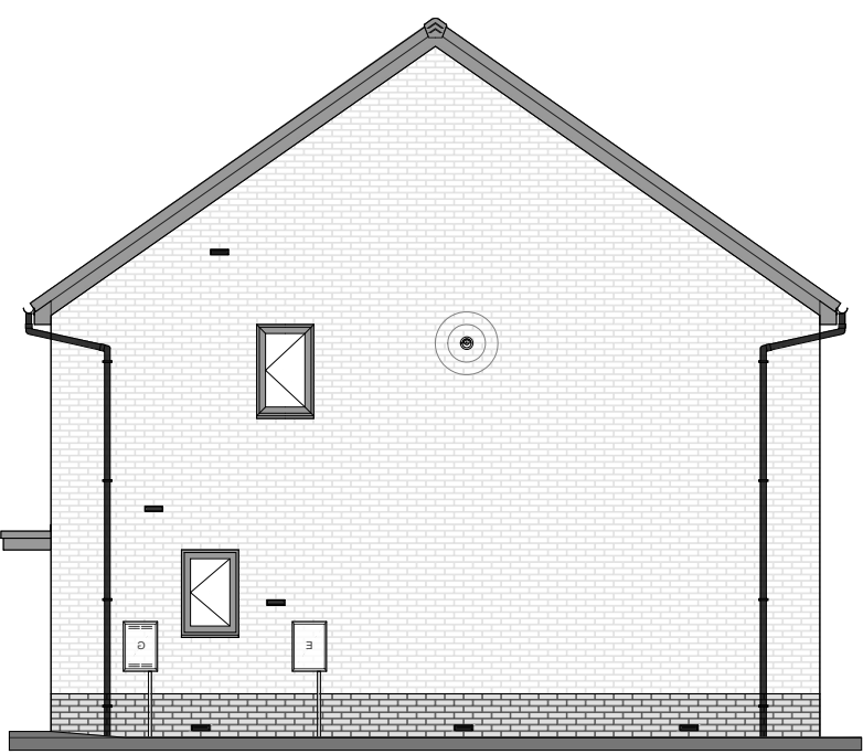
RIGHT ELEVATION
