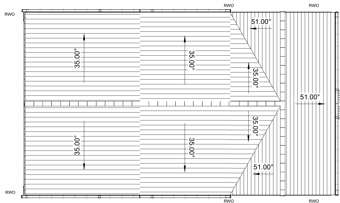
Roof Plan 1 : 100
