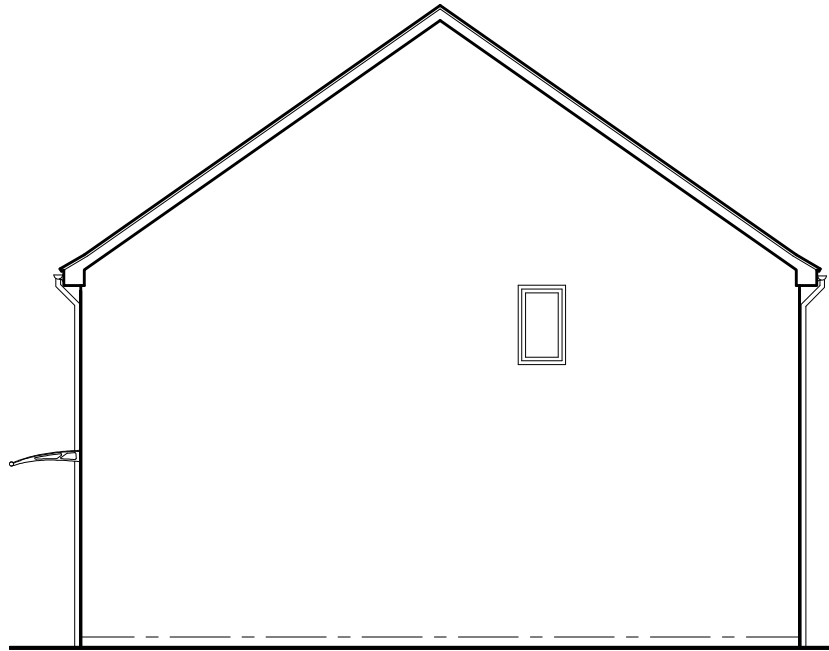
Side Elevation (opp)
