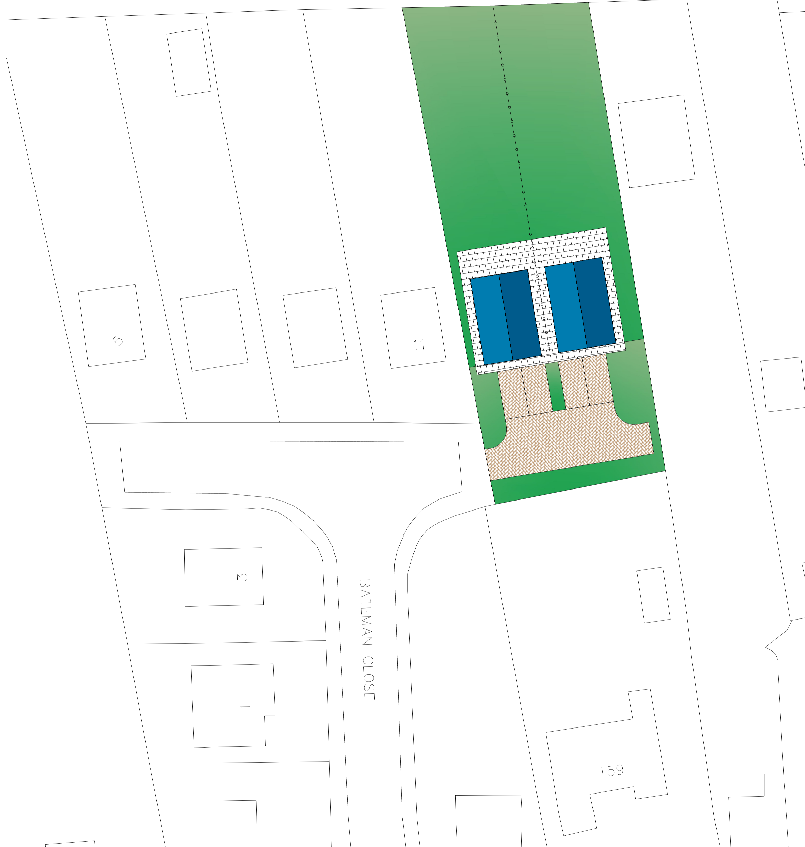
SITE PLAN 1:200
