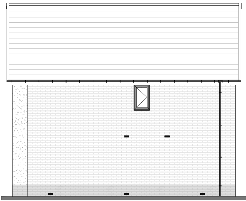
RIGHT ELEVATION
