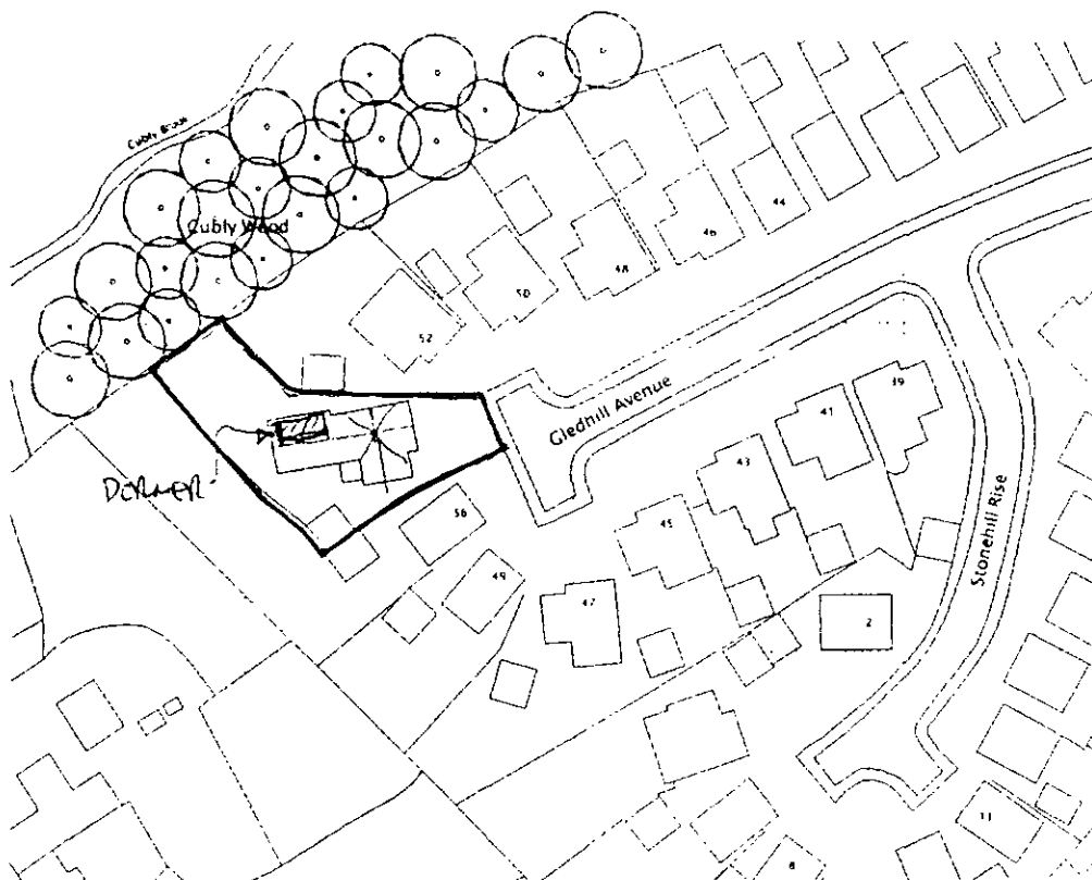
Site Plan - 1:500
