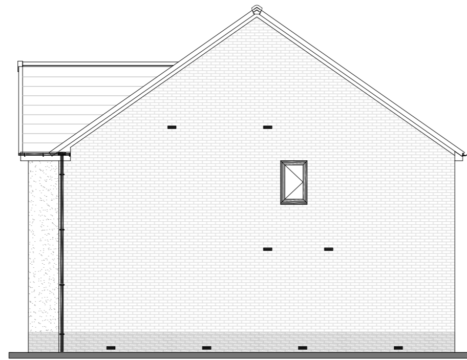
RIGHT ELEVATION
