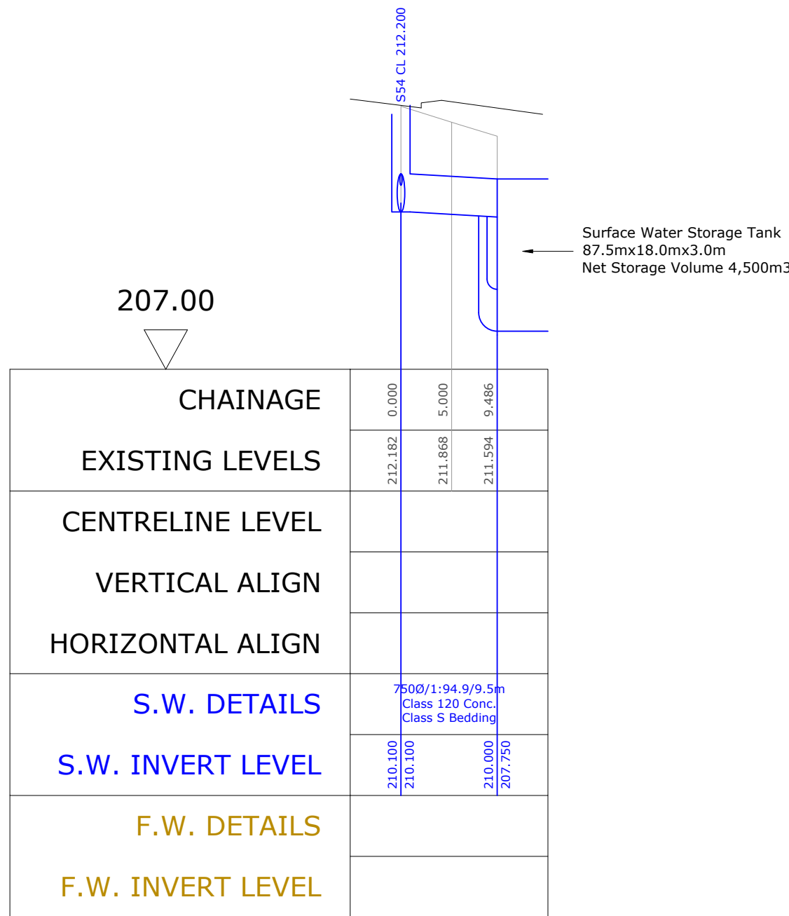
S54-T2 Horiz. 1:500 Vert. 1:100
