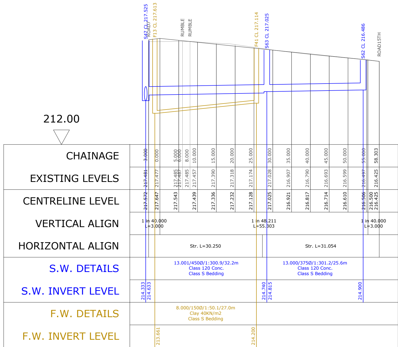
ROAD15 Horiz. 1:500 Vert. 1:100
