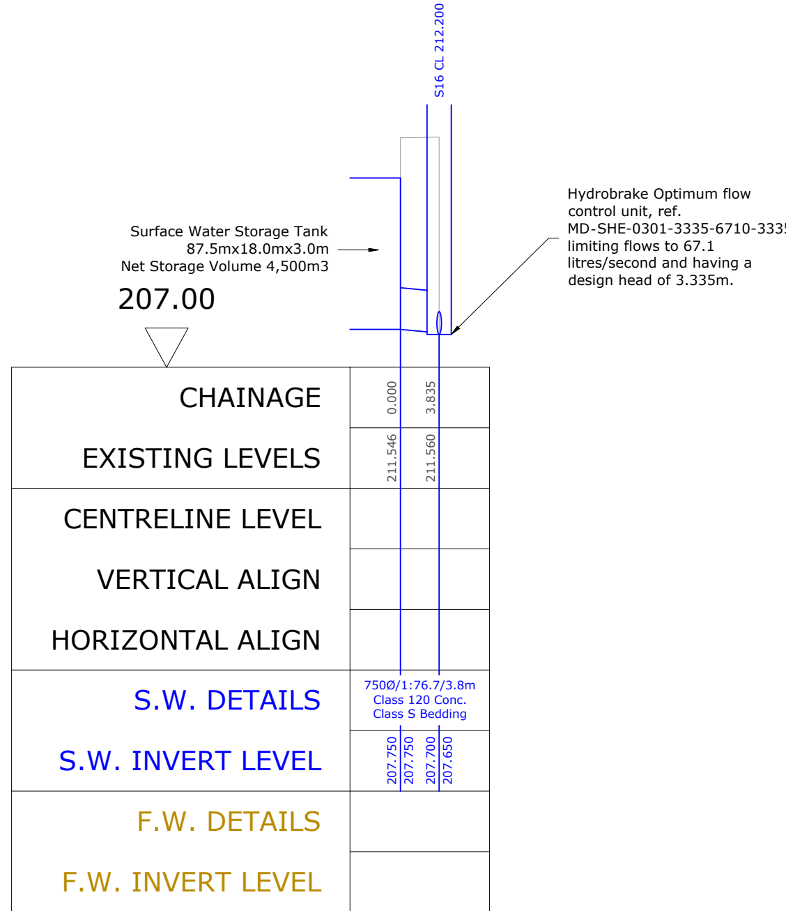
T3-S16 Horiz. 1:500 Vert. 1:100
