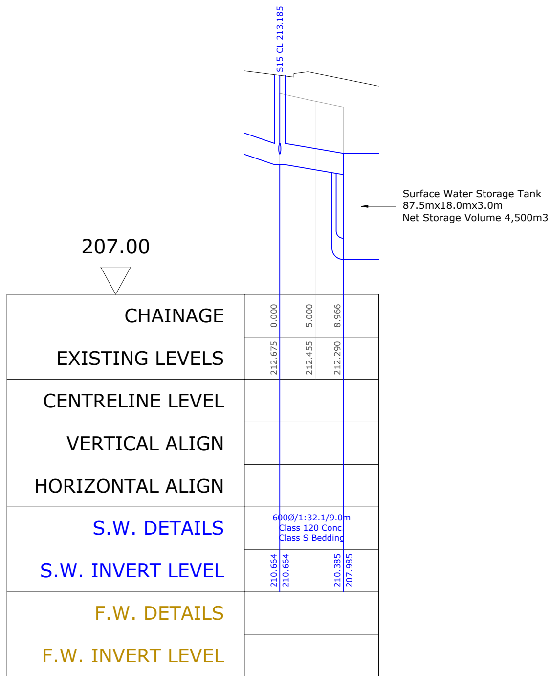
S15-T1 Horiz. 1:500 Vert. 1:100
