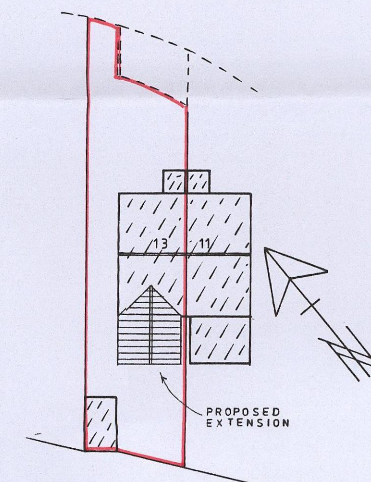
SITE PLAN 1:250
