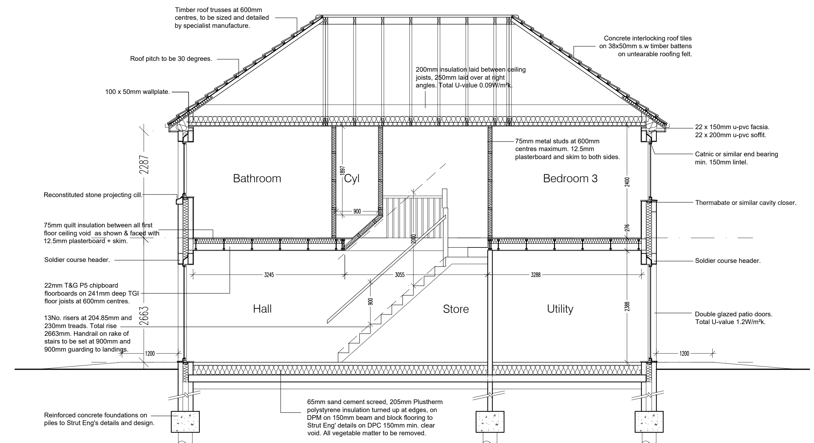
Section A-A
