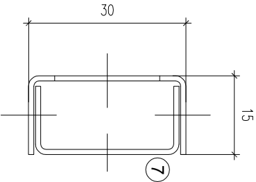
WIRING BAR Scale 1:1
