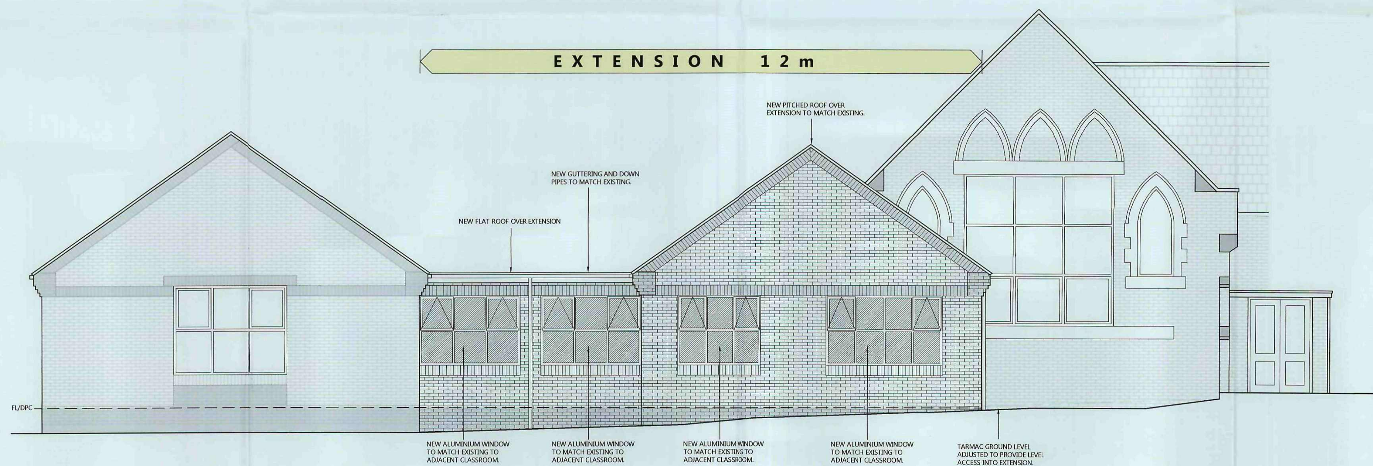
ELEVATION B
