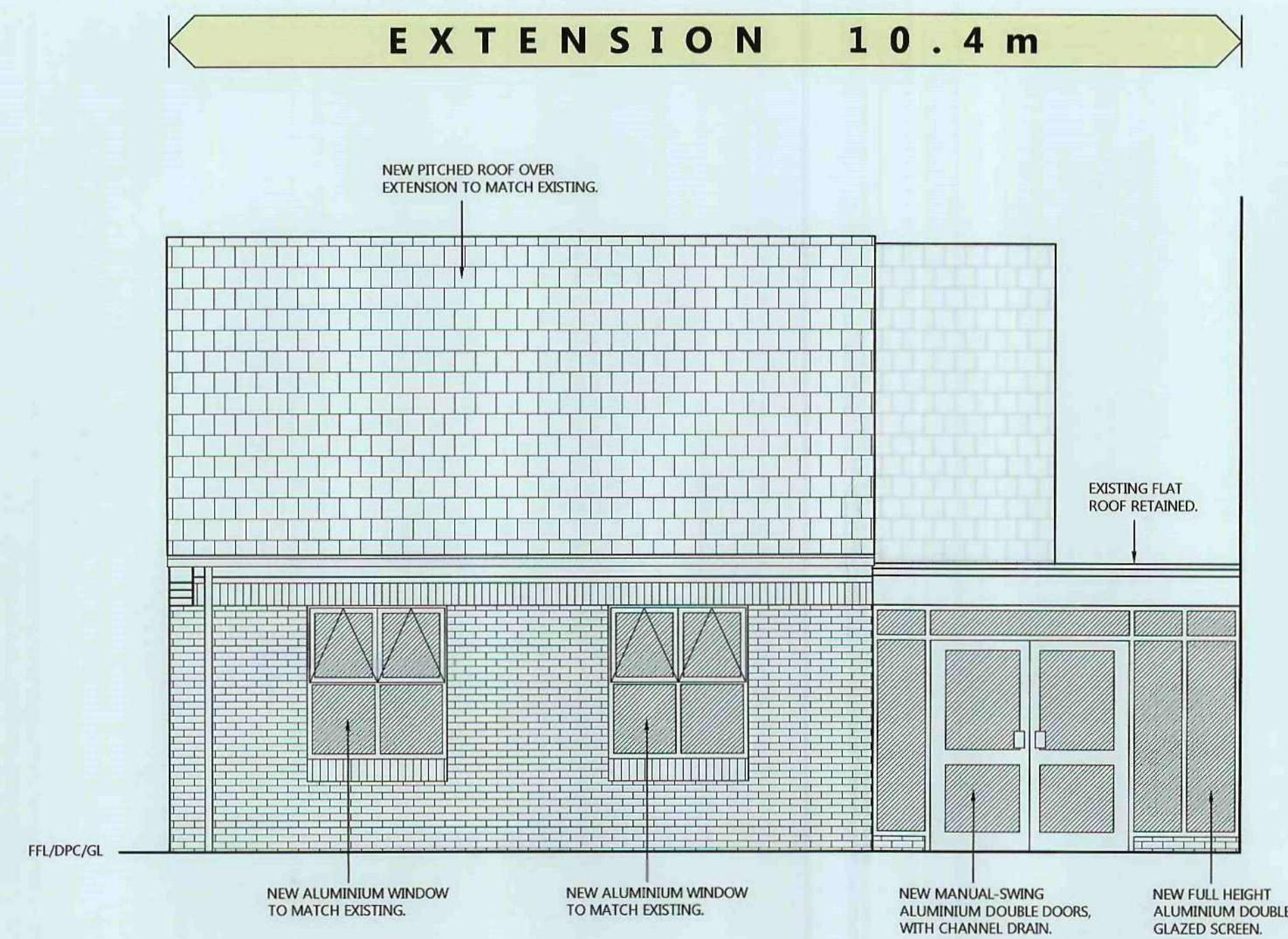
ELEVATION A
