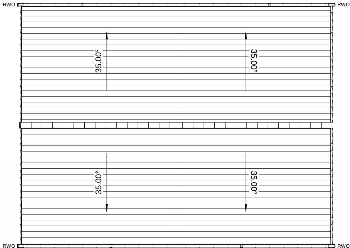
Roof Plan 1 : 100
