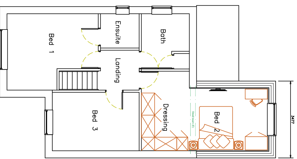
F.F. Plan
