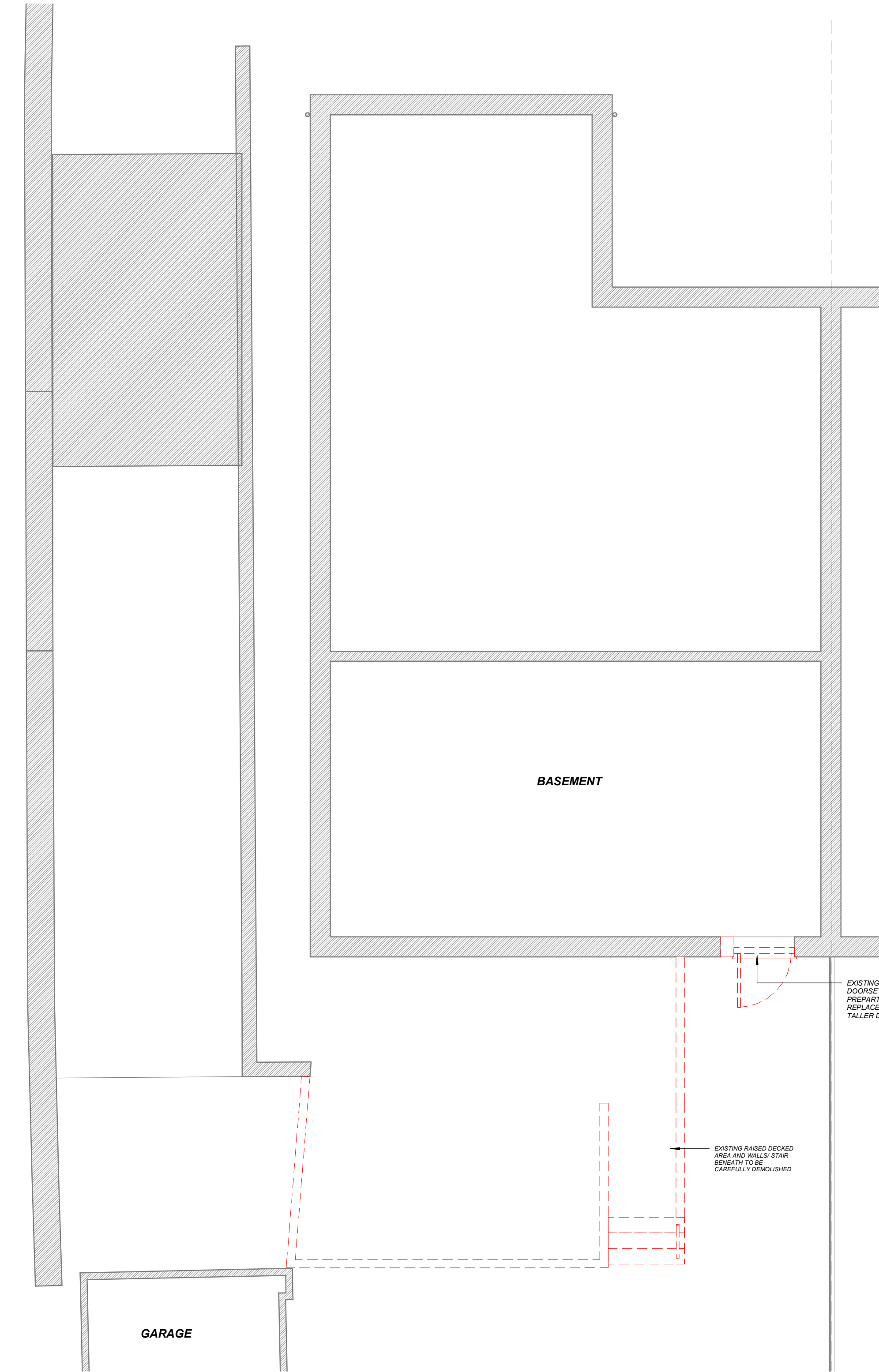
EXISTING BASEMENT GA PLAN 1 : 50
