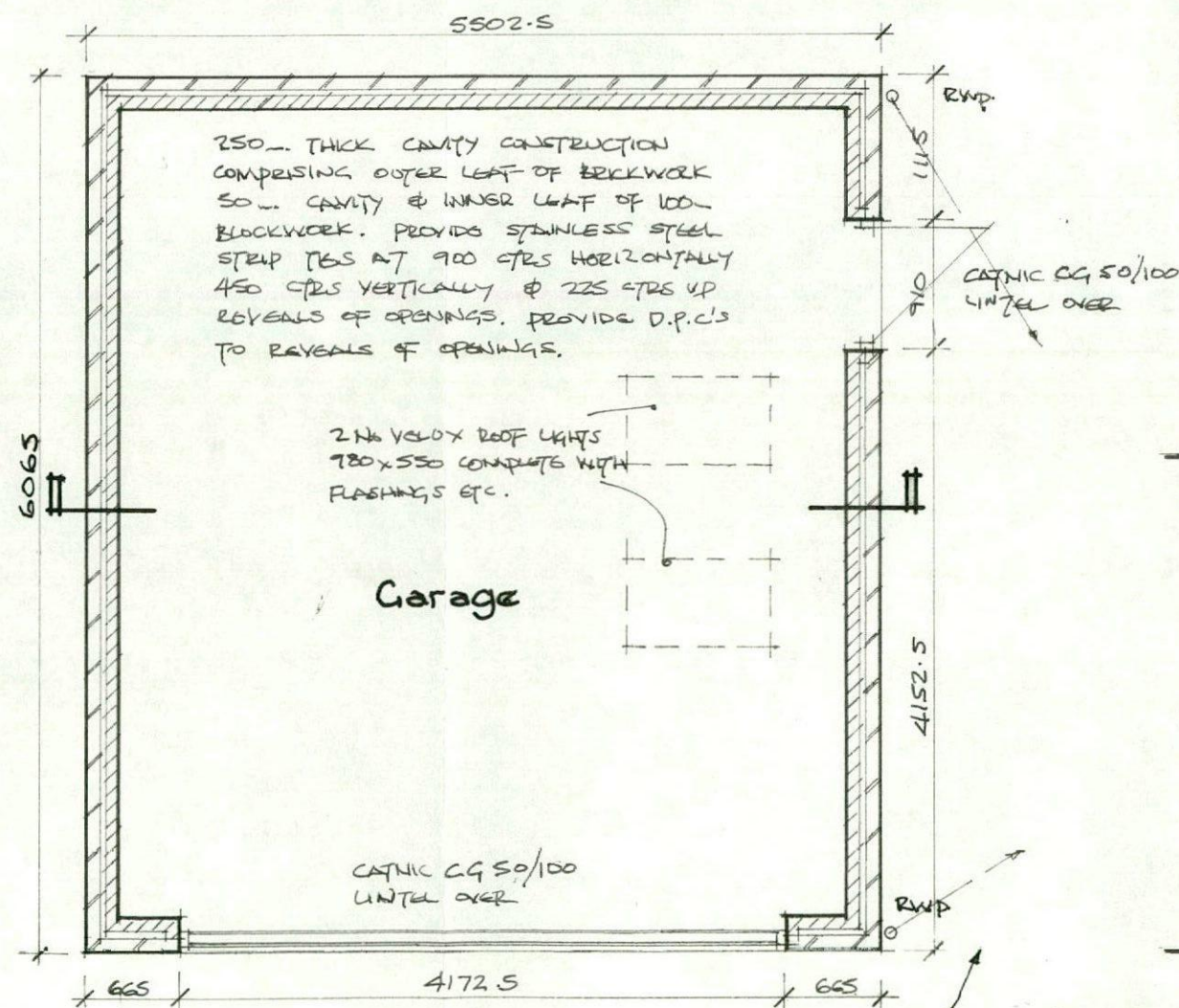
PLAN 1:50
