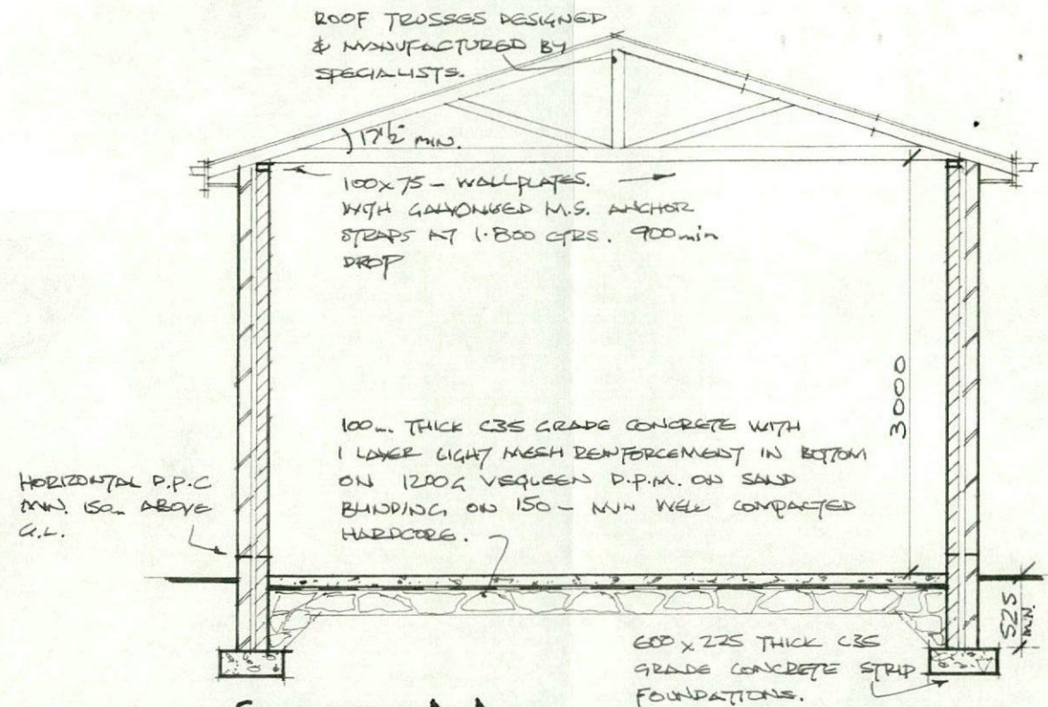
SECTION A-A 1:50
