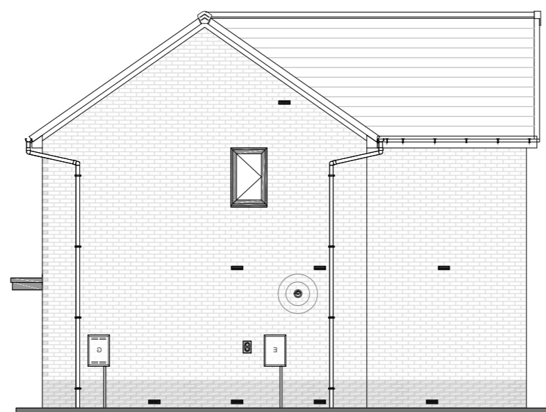
RIGHT ELEVATION
