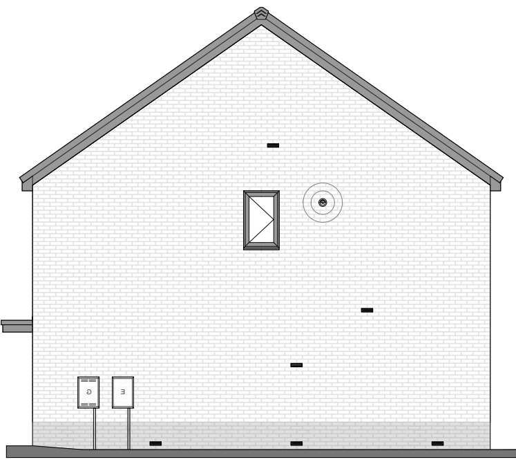
RIGHT ELEVATION
