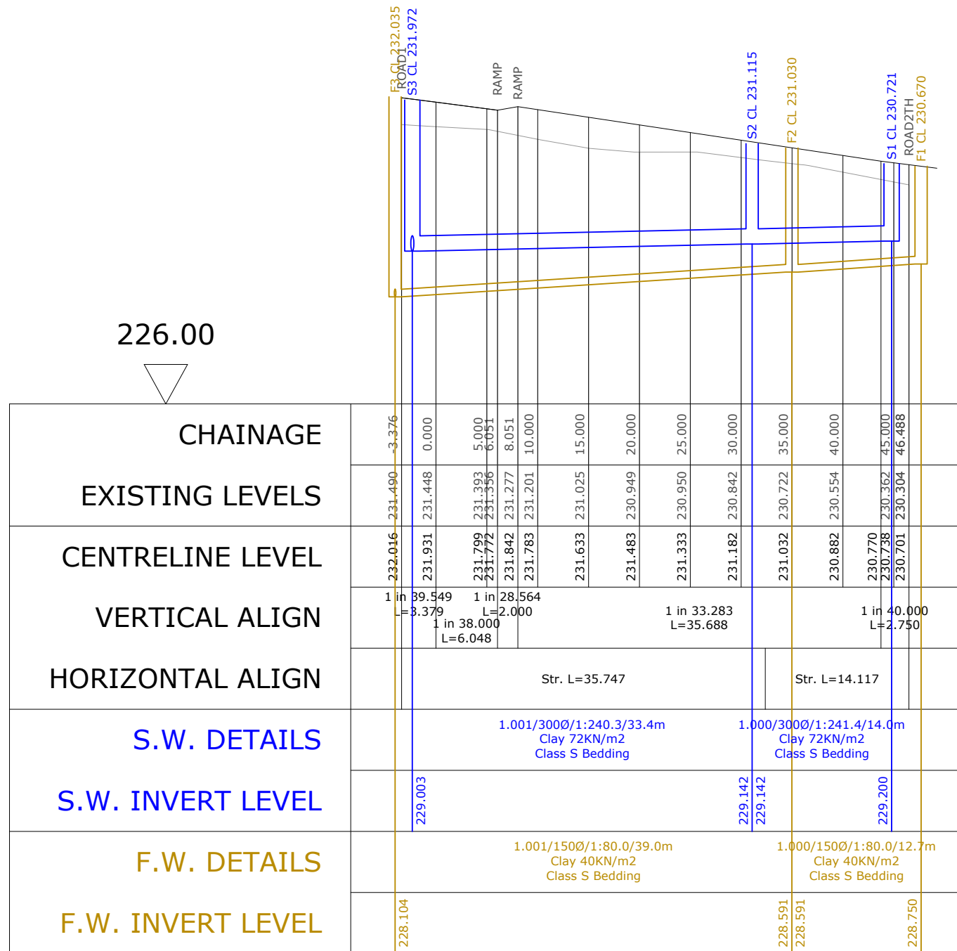
ROAD1 Horiz. 1:500 Vert. 1:100
