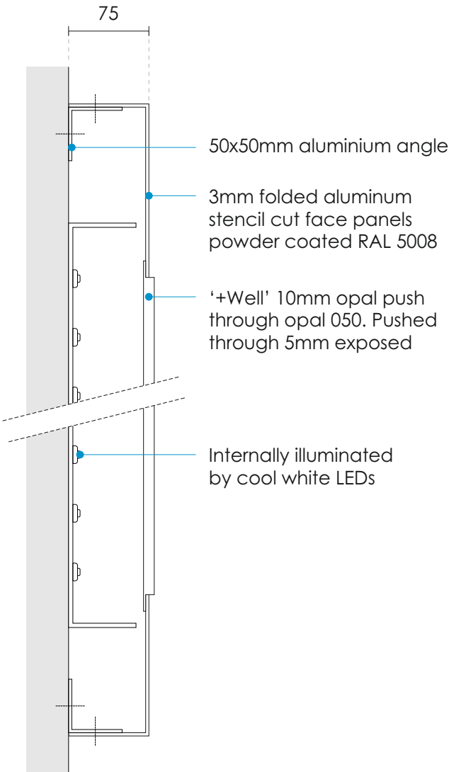
'+well' section 1:5@A3
