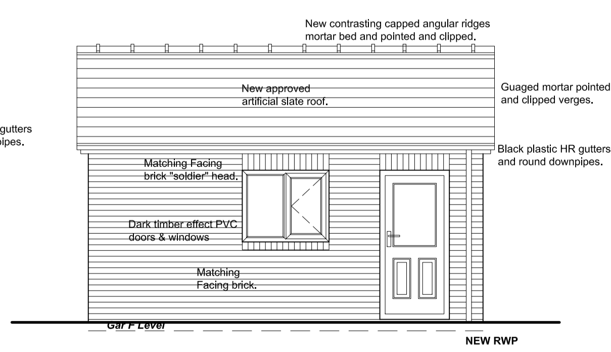
SIDE ELEV R
