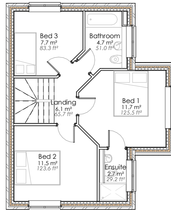
2 | *L01 - HTG 1 : 100
