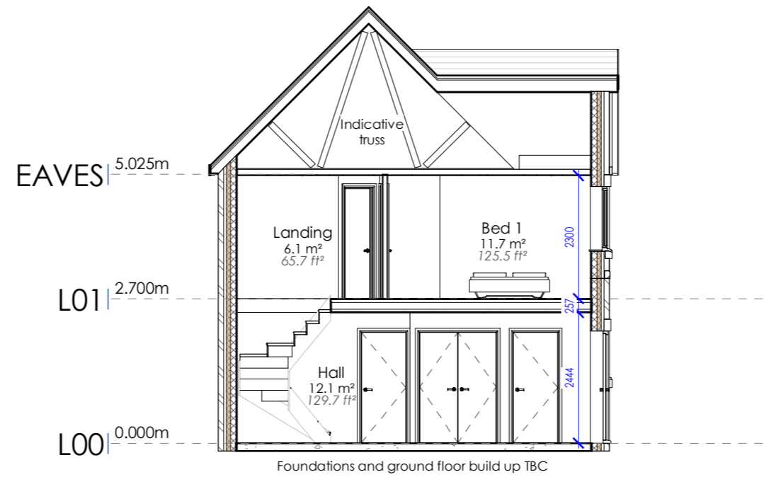
7 | HTG Section 1 : 100
