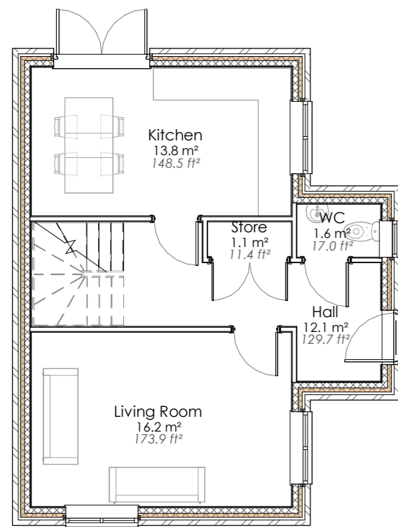
1 | *L00 - HTG 1 : 100
