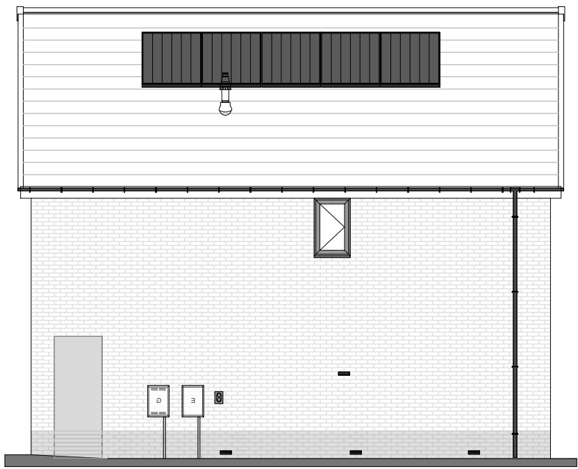
RIGHT ELEVATION
