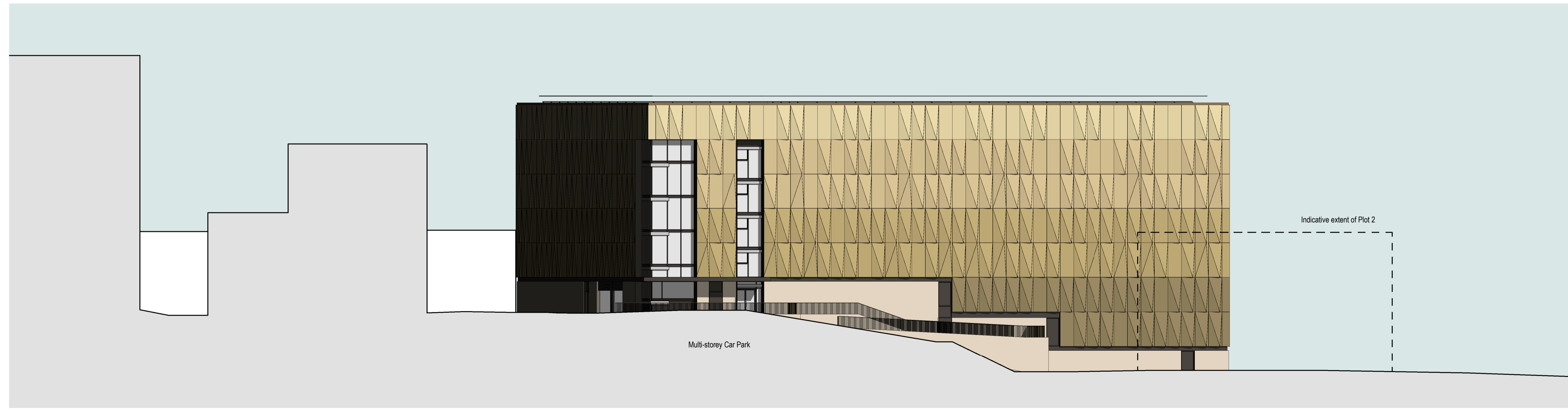
2 MSCP Site Cross Section 2 1 : 200
