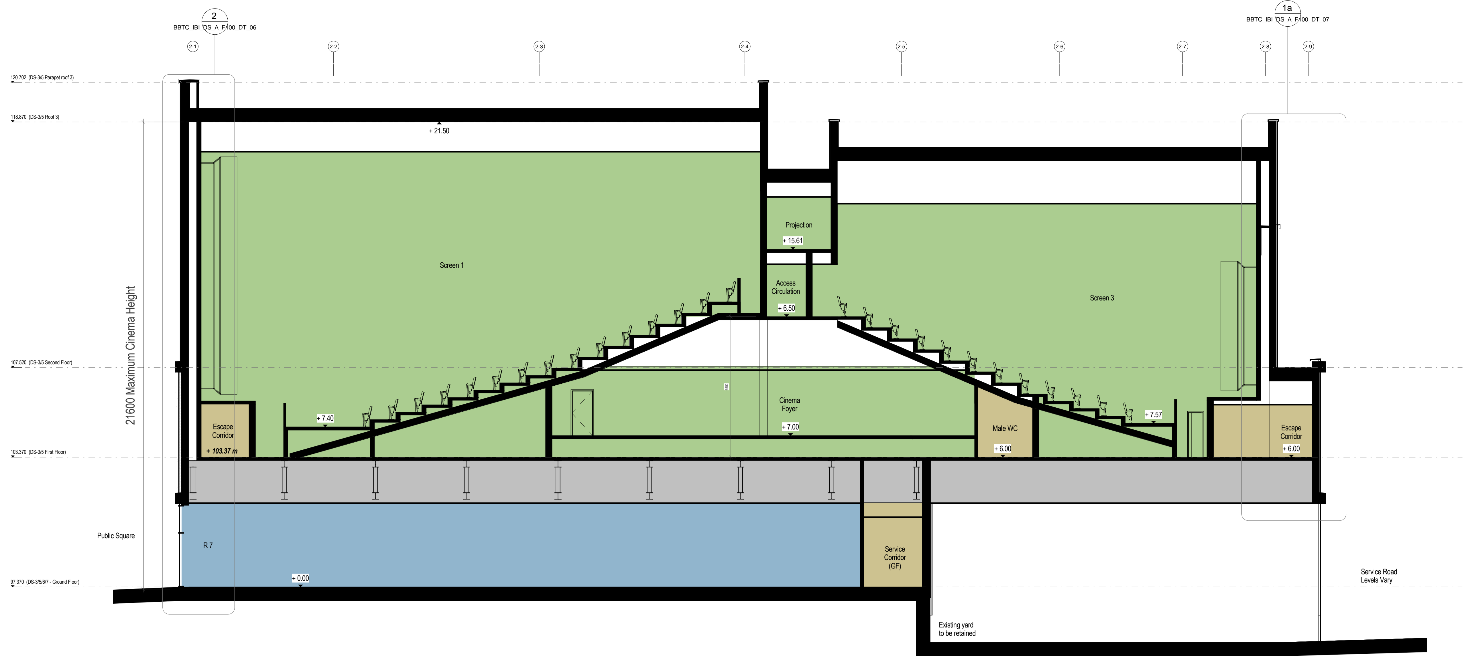
A1 Section A1 1:100
