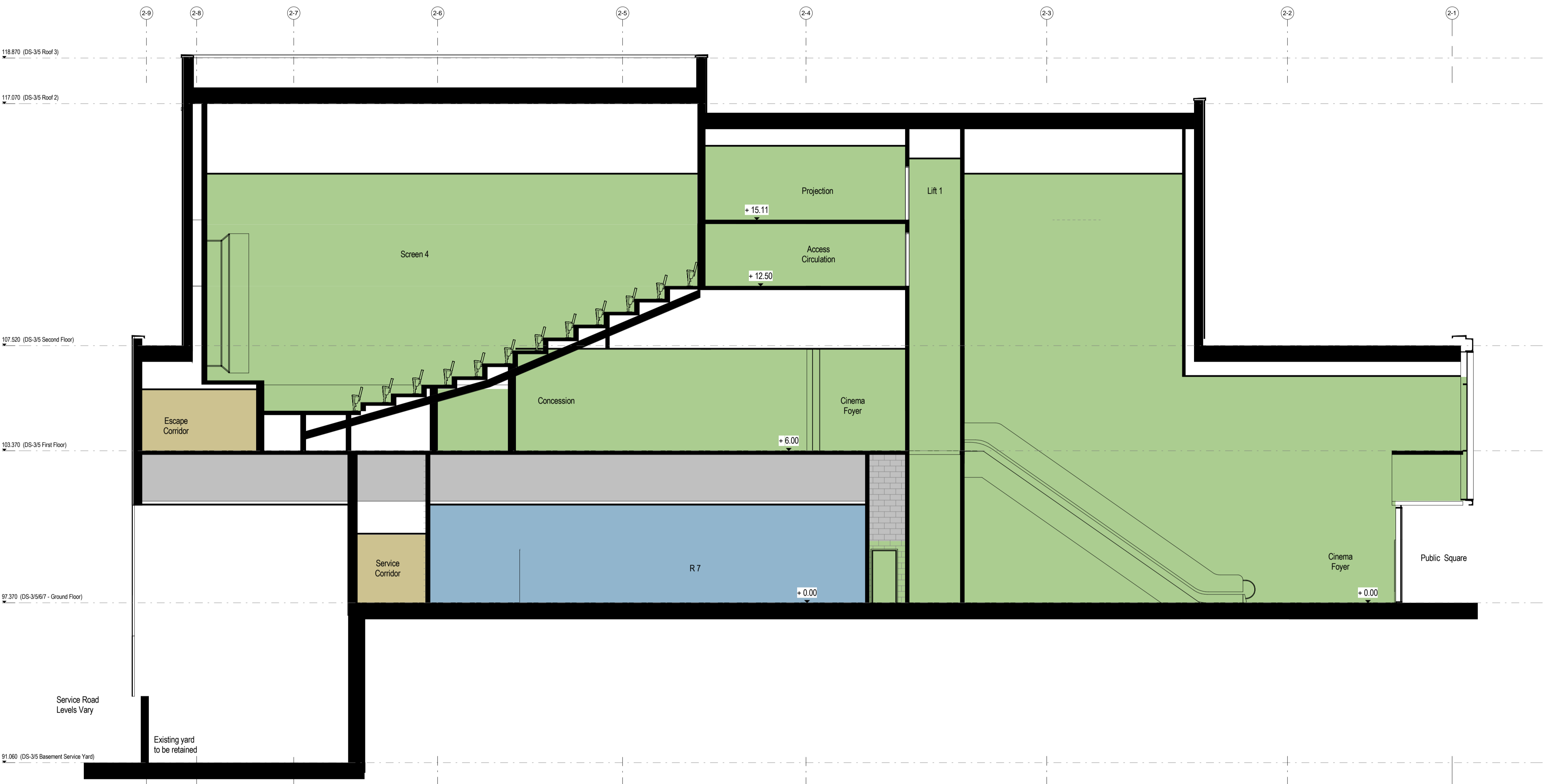
A2 Section A2 1:100
